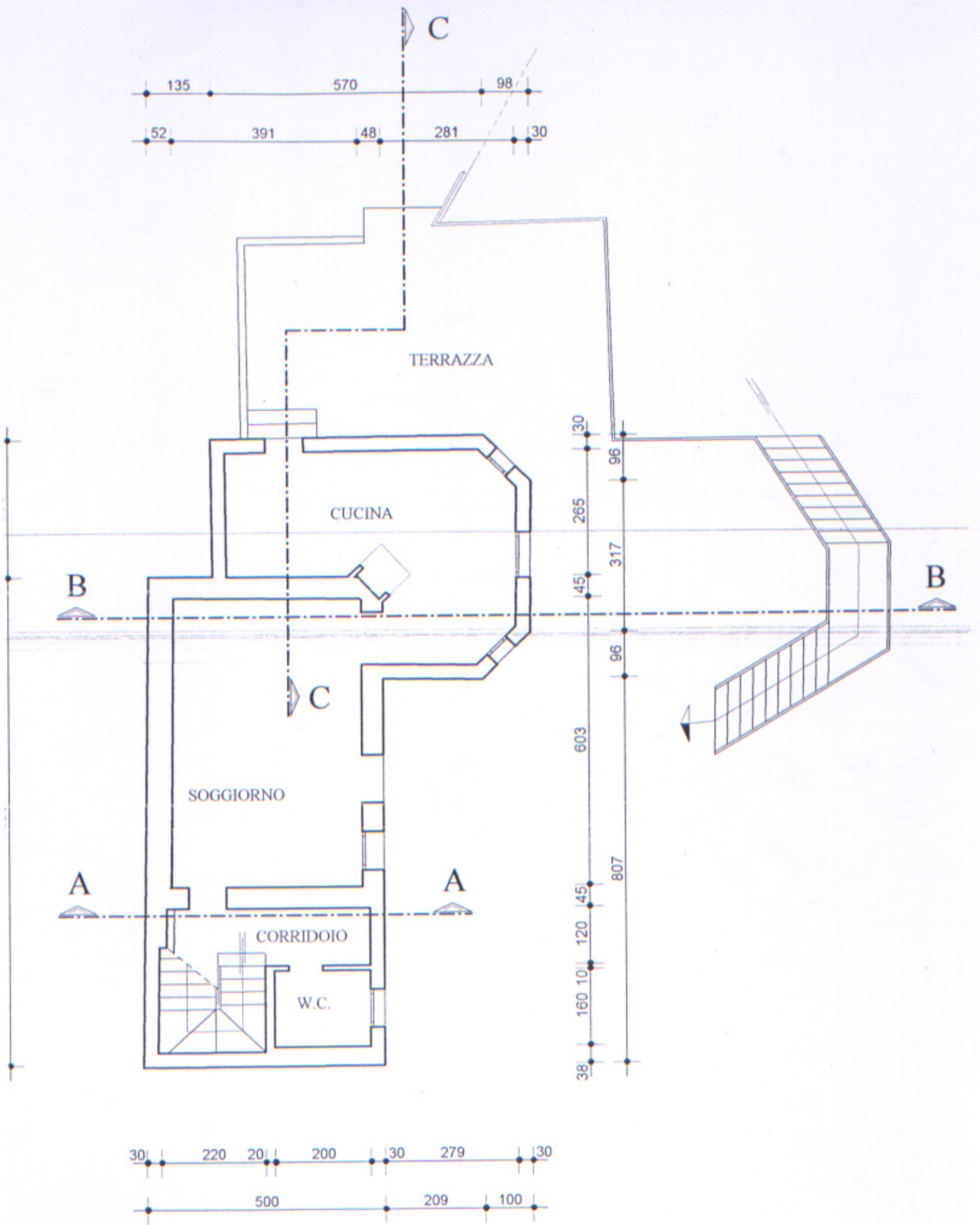
PIANTA 2° LIVELLO
